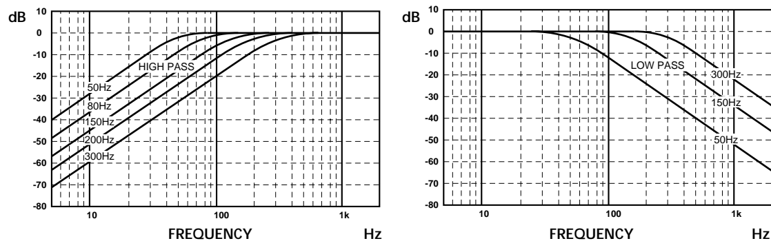
Cut-off frequency/Fréquence de coupure
