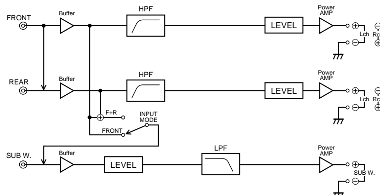
Circuit Diagram/Schéma du circuit
